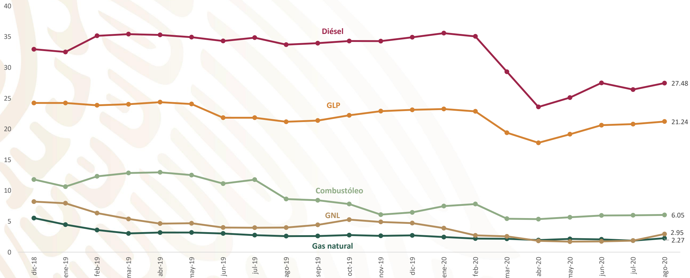
Precios de combustibles (USD/MMBTU)
