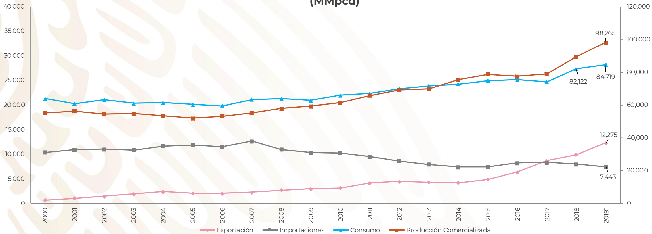
Producción, consumo, importación y exportación de gas natural en Estados Unidos (MMpcd)
